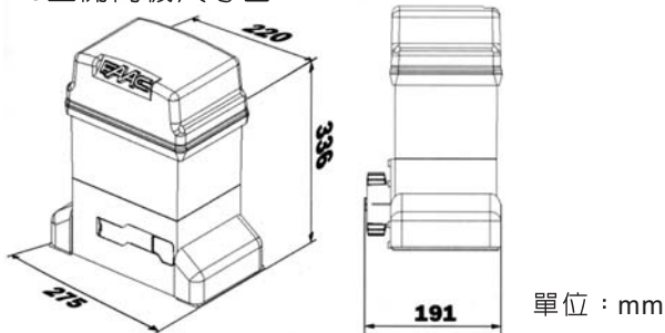
746型開門機尺寸圖
